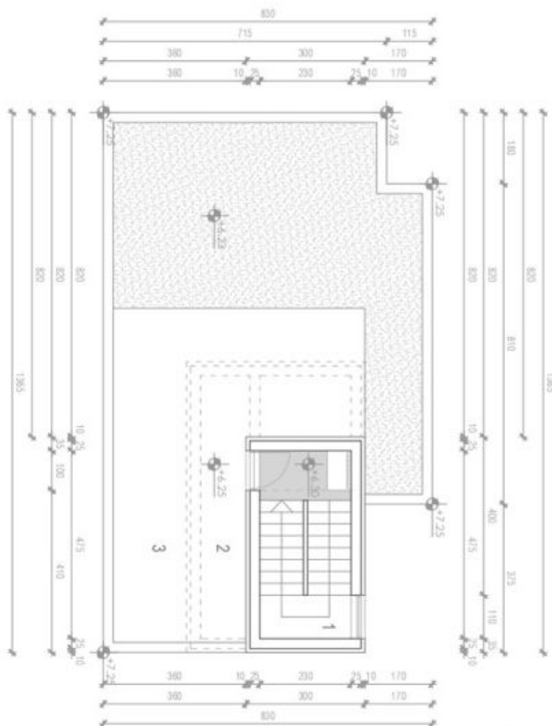
TLOCRTI KROVNE TERASE
