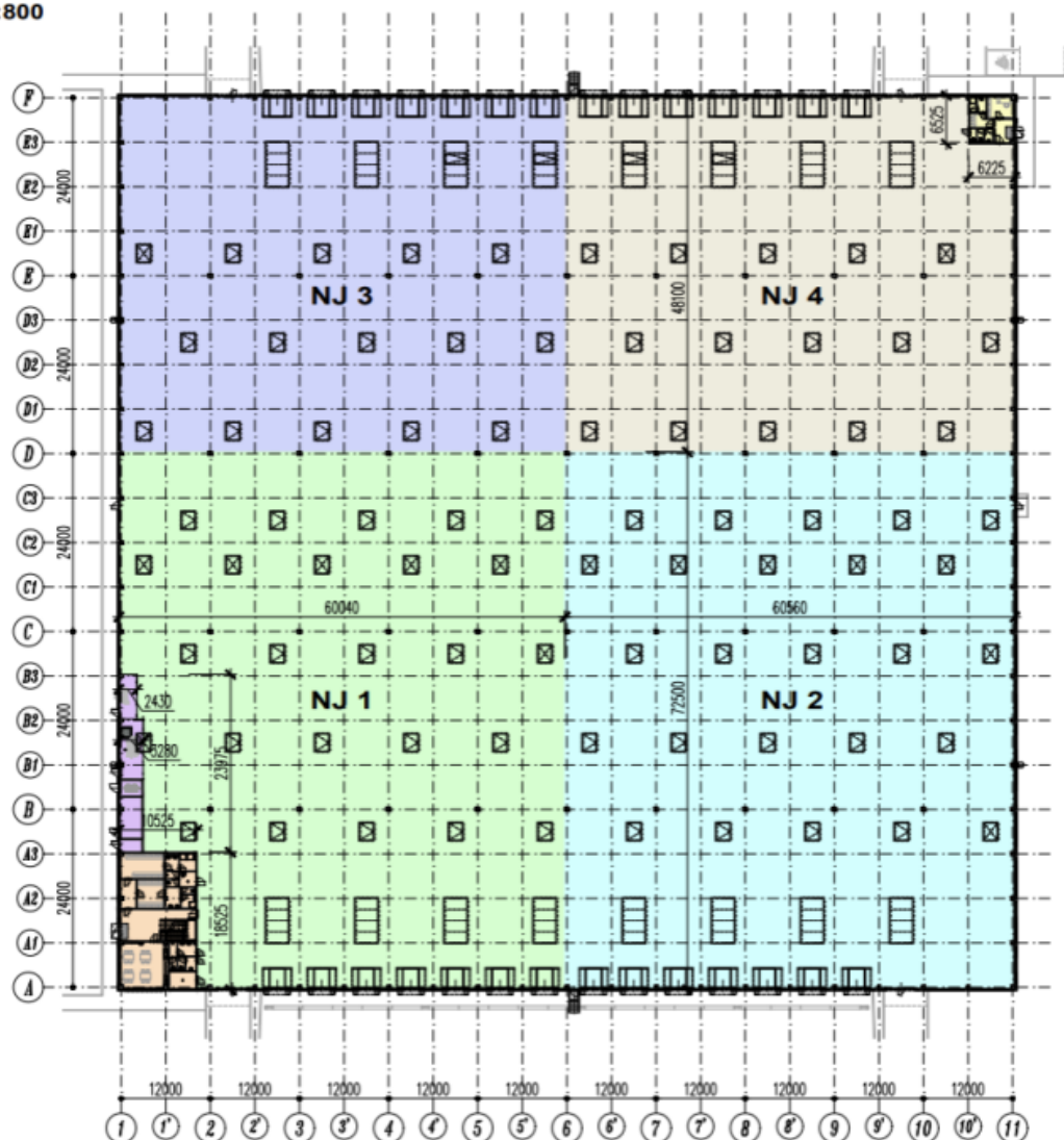
PŮDORYS 1.NP 1:800
