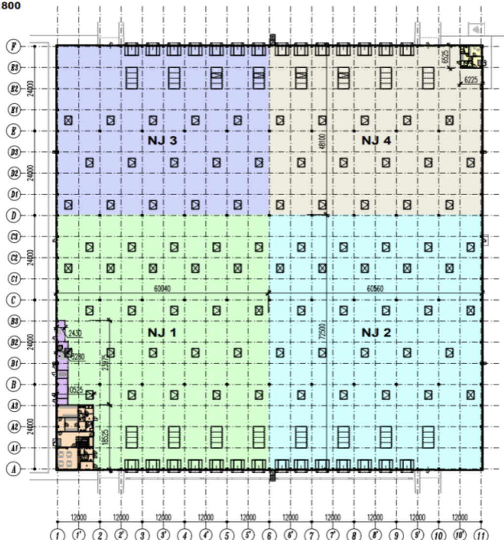
PŮDORYS 1.NP 1:800
