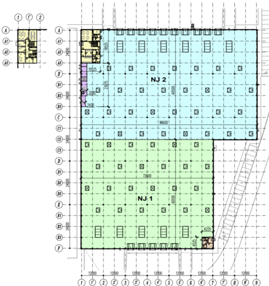
PŮDORYS 2.NP 1:800
