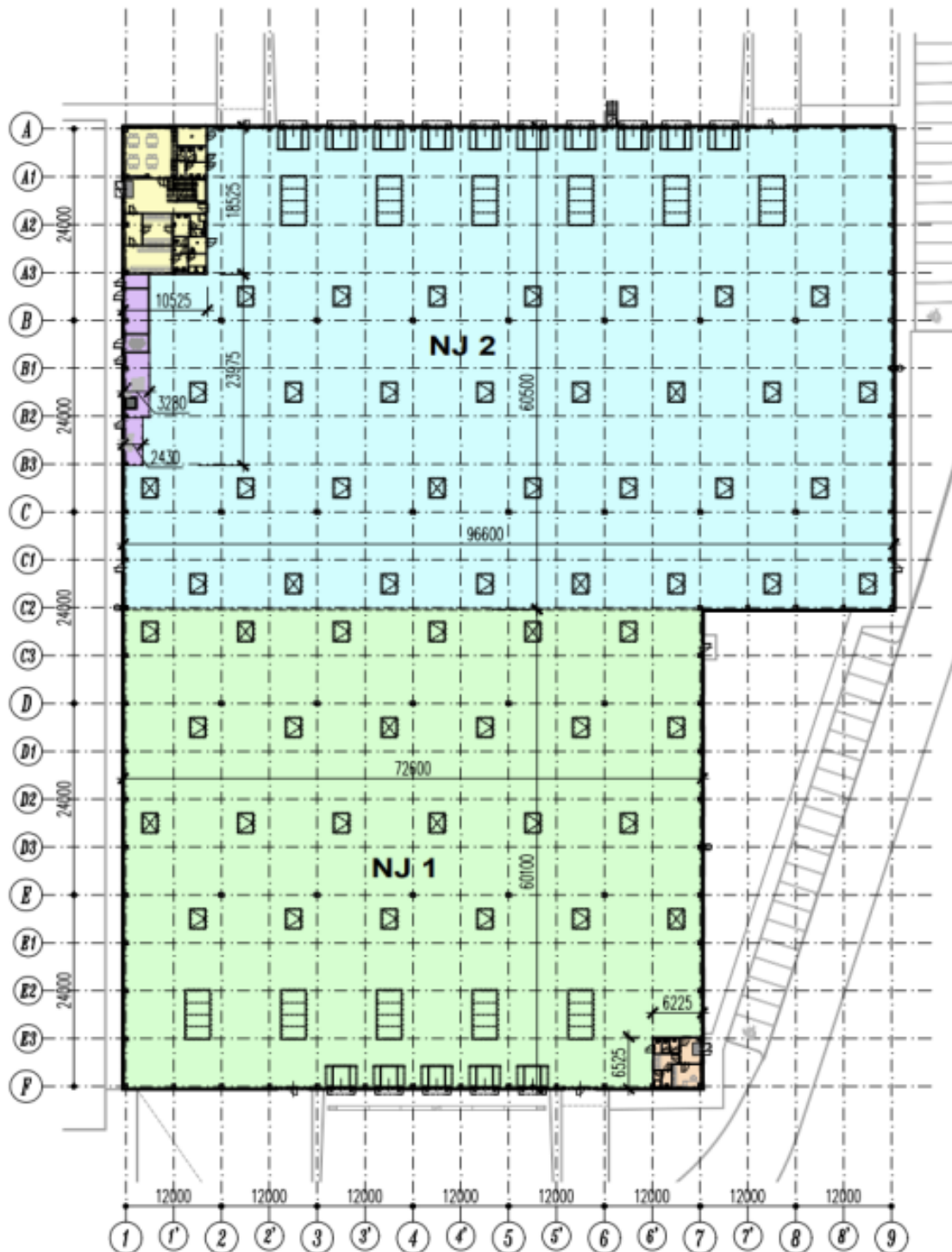
PŮDORYS 1.NP 1:800
