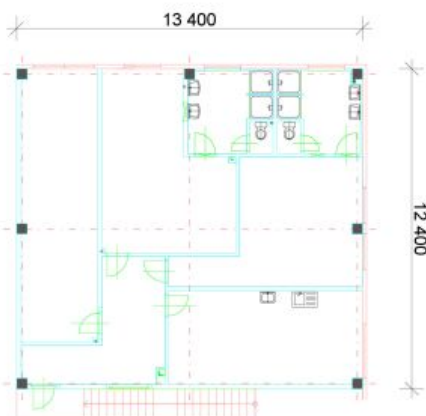
PŮDORYS 2.NP
