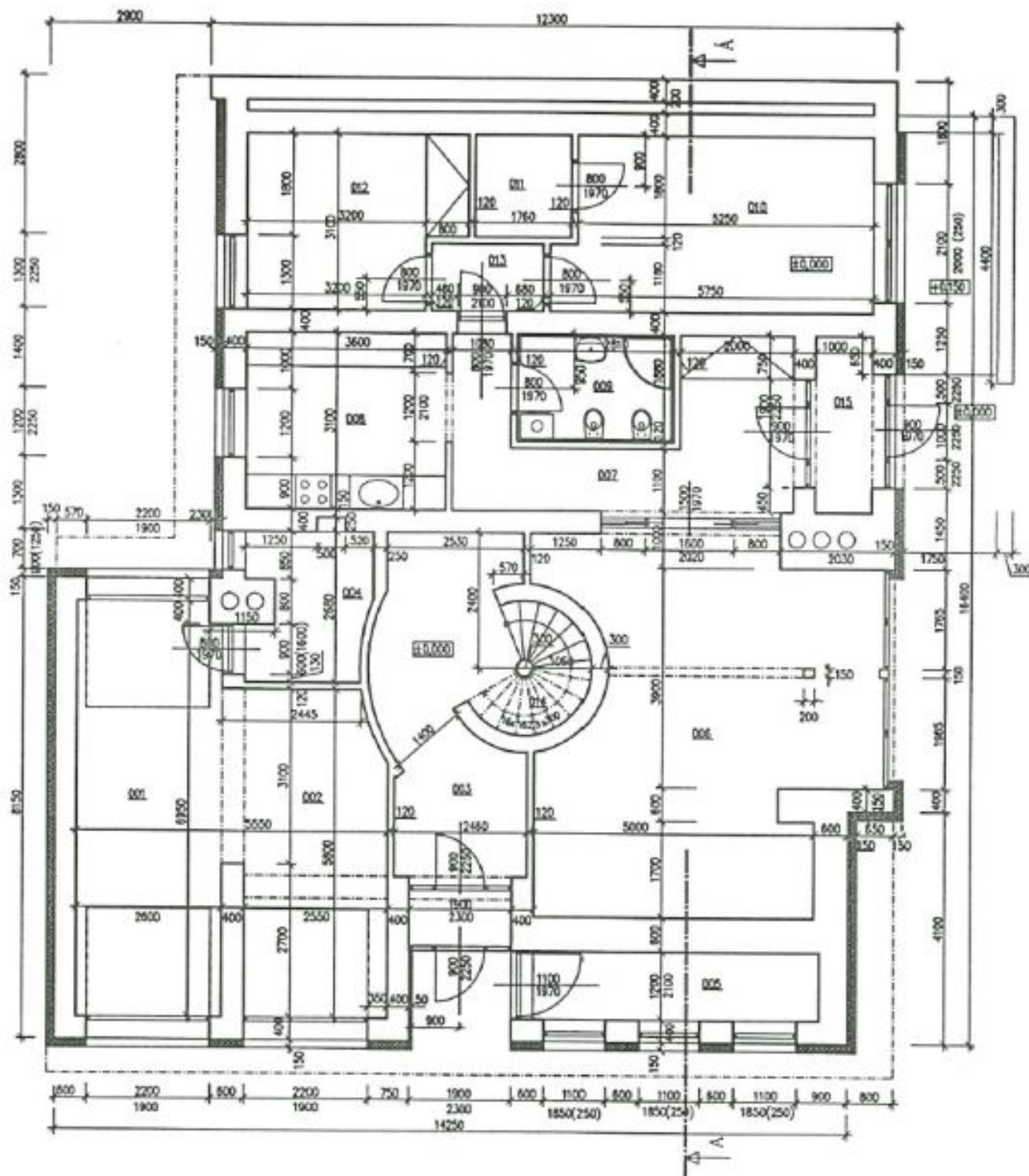
PŮDORYS I.PP
