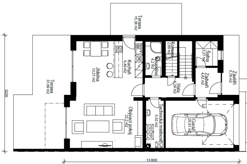
PŮDORYS 1.NP
