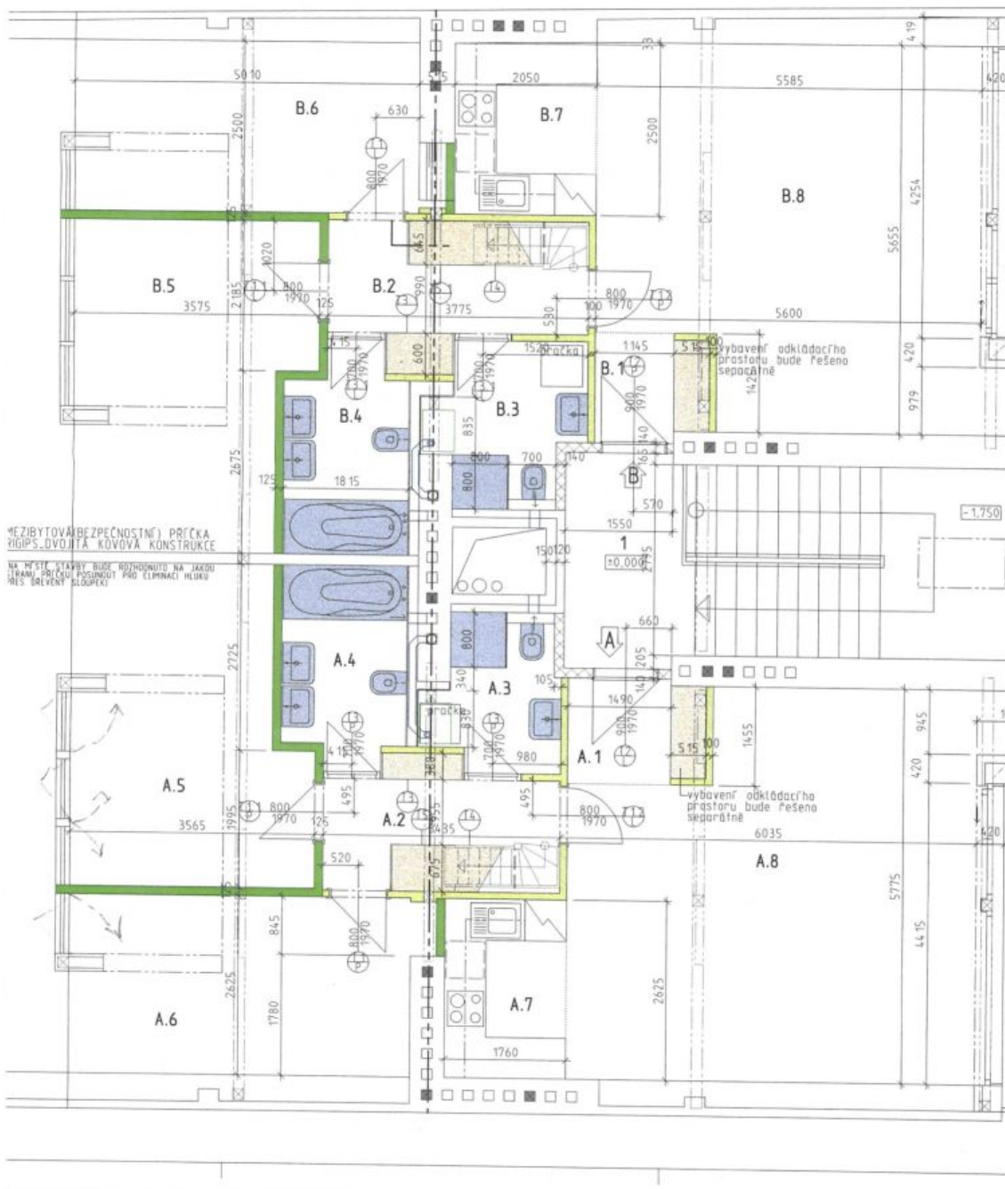
RYŠ PODKROVÍ, 1/50
