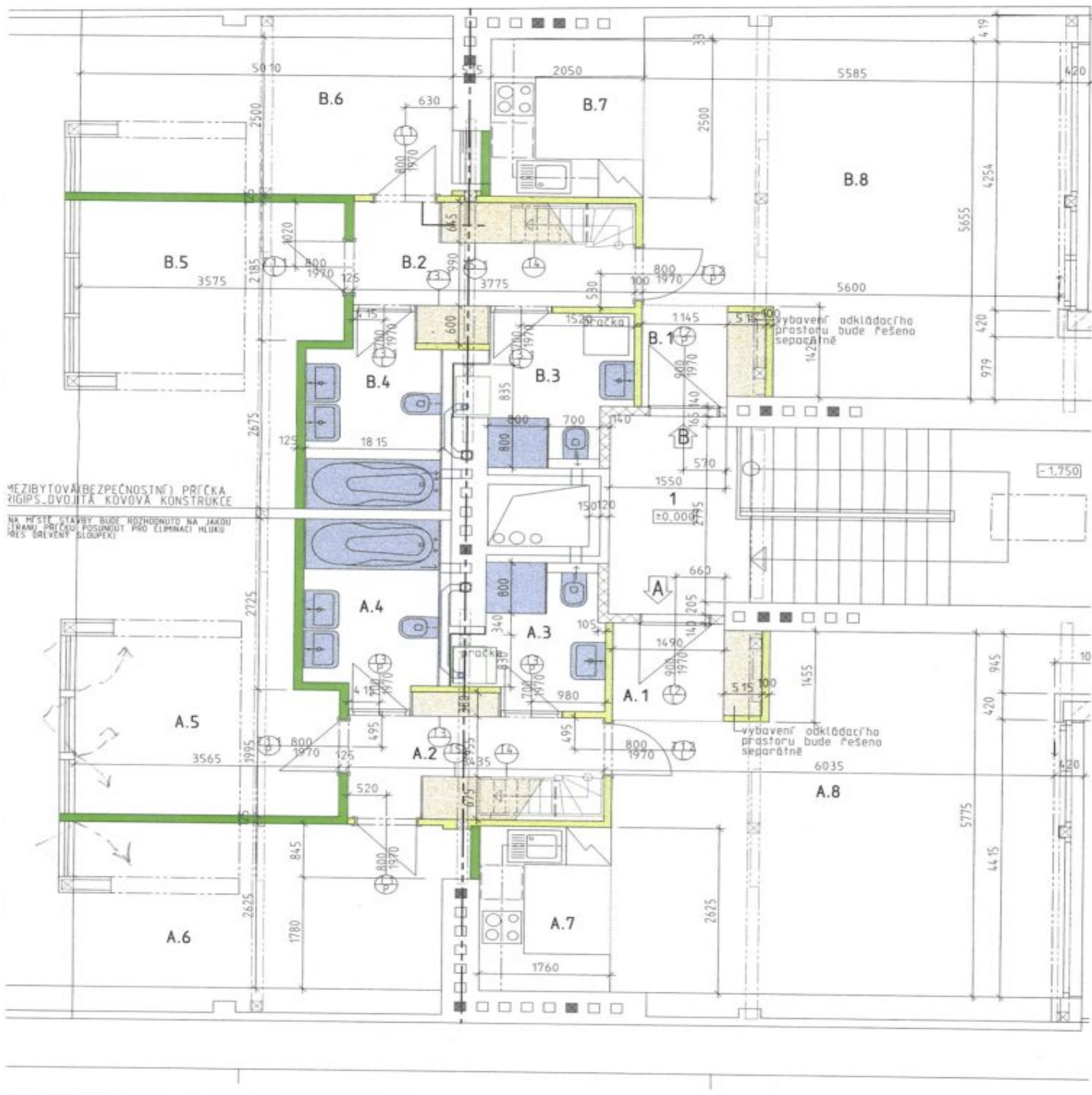
RYŠ PODKROVÍ, 1/50
