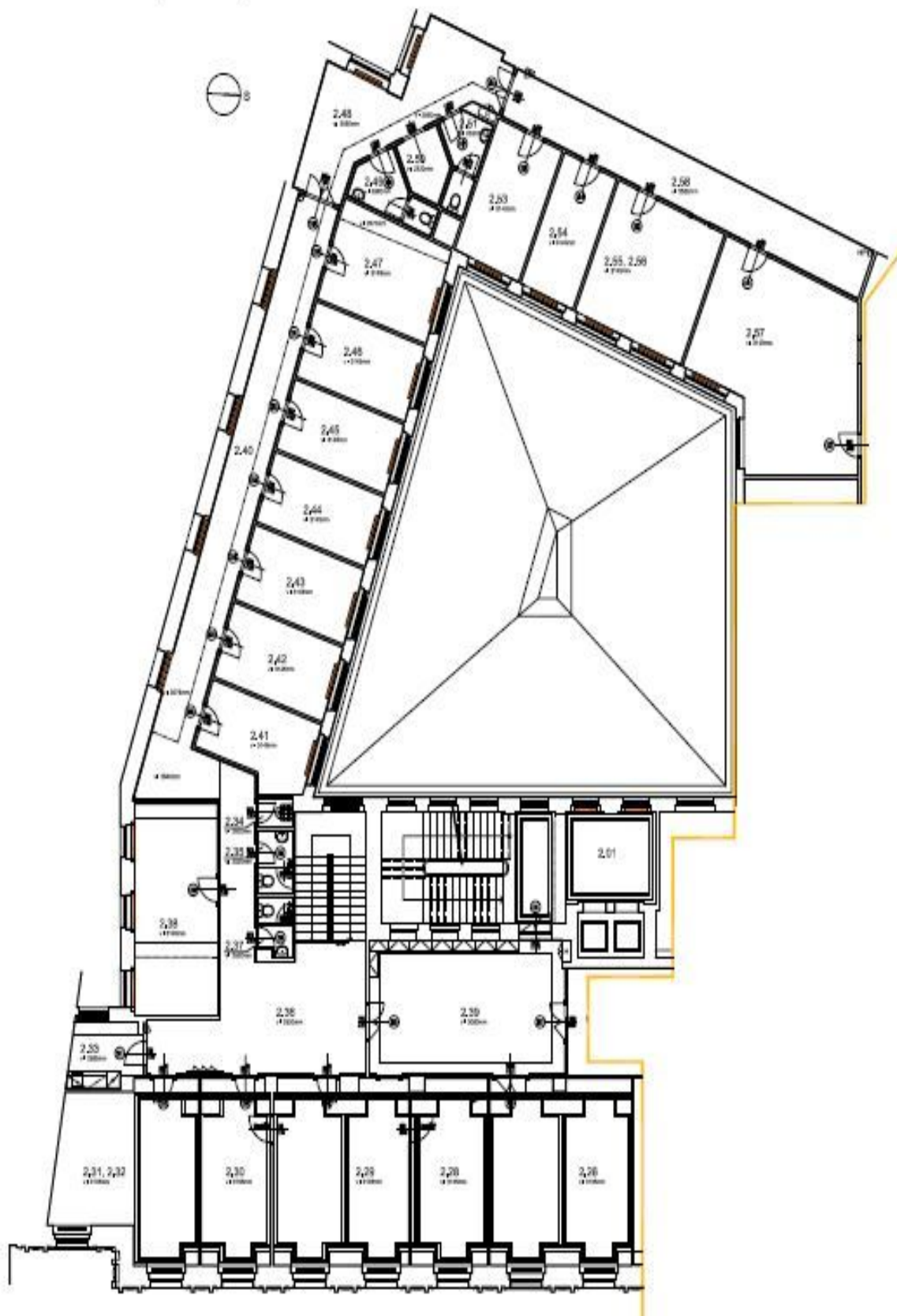
PŮDORYS 4.NP (2.PATRO) M 1:100
