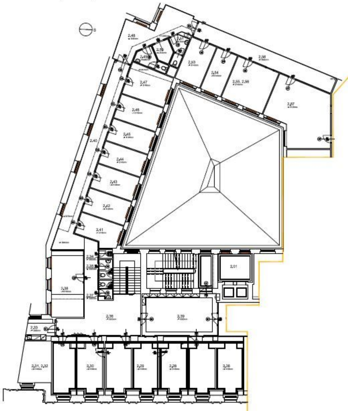
PŮDORYS 4.NP (2.PATRO) M 1:100
