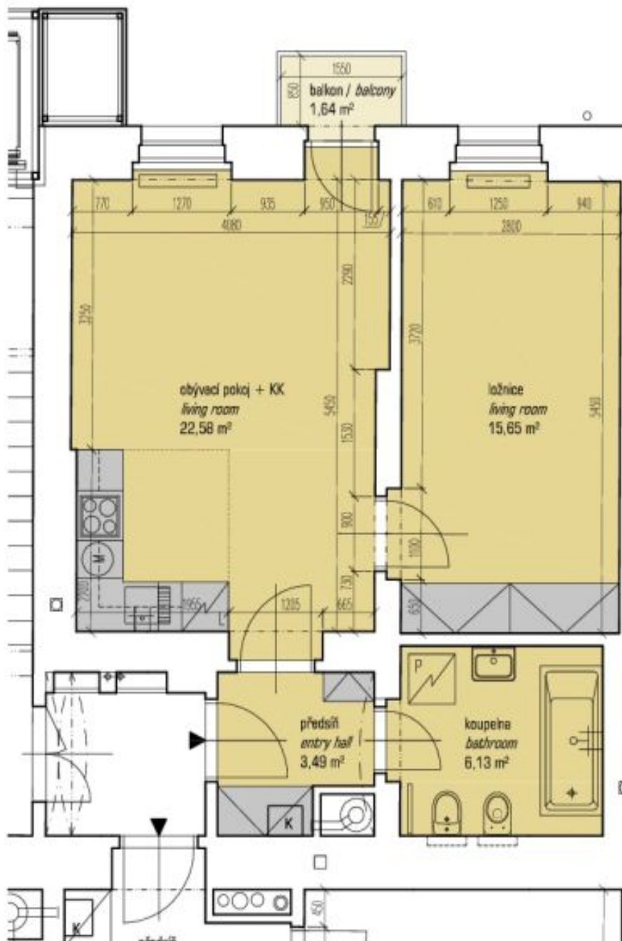
byt č. 5 / flat n. 5 / 3.NP / 49,49 m 2
