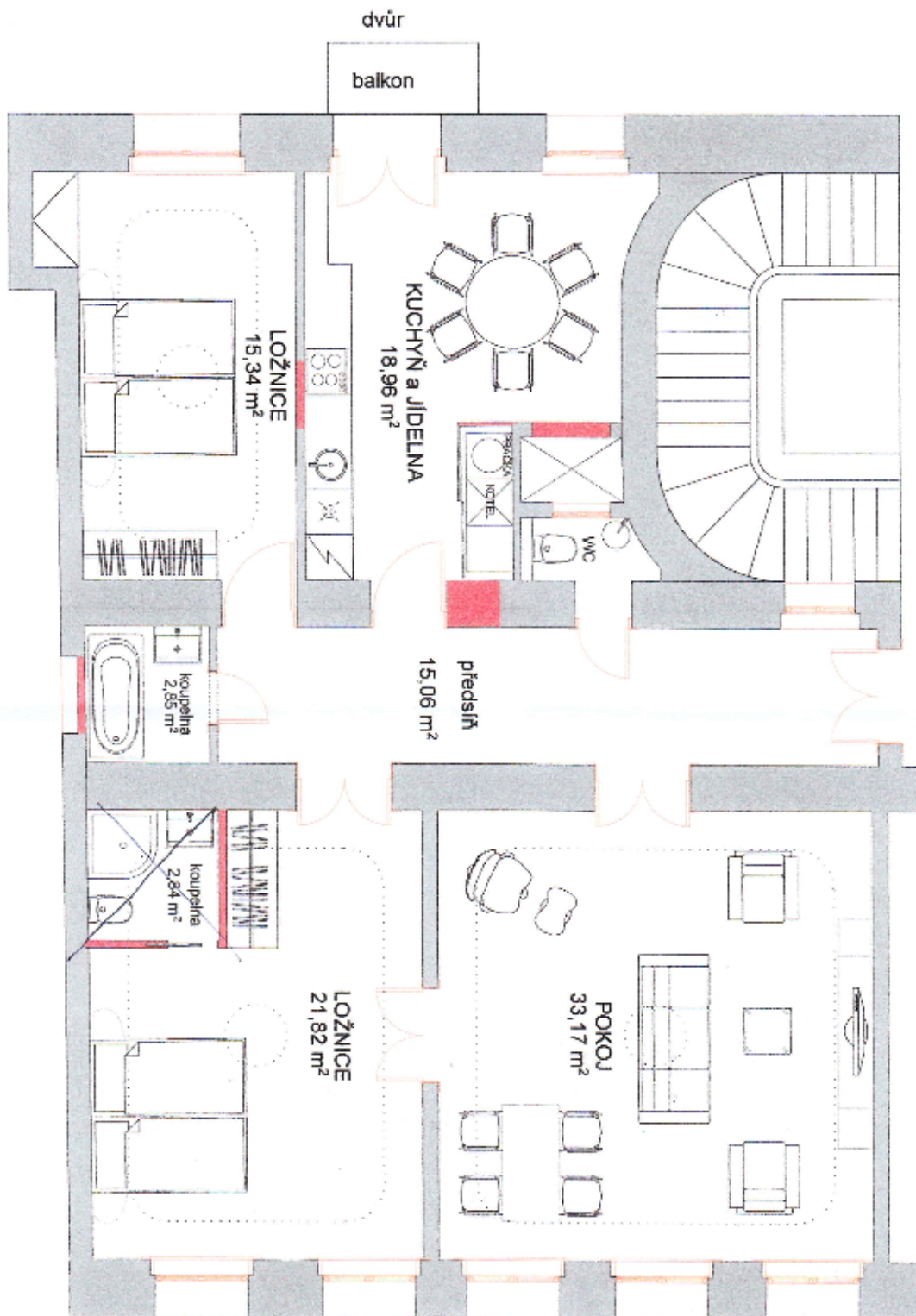
BYT VE 2.PATŘE DOMU Č.67/11 V PLASKÉ ULICI, PRAHA 5 VARIANTA D
