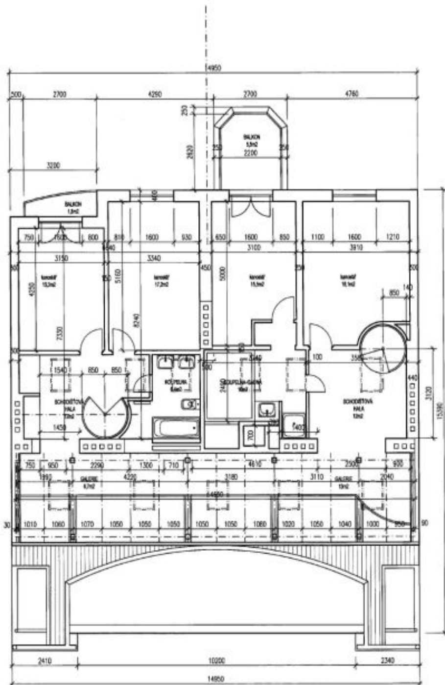
Půdorys 6.NP
