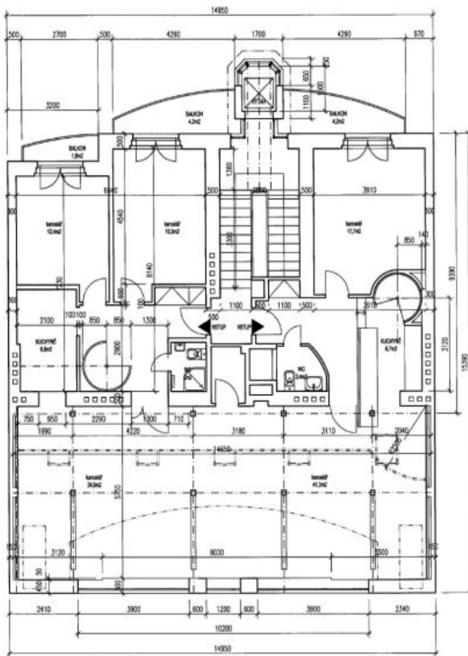
Půdorys 5.NP
