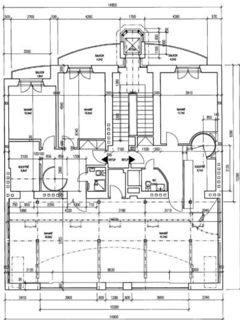
Půdorys 5.NP
