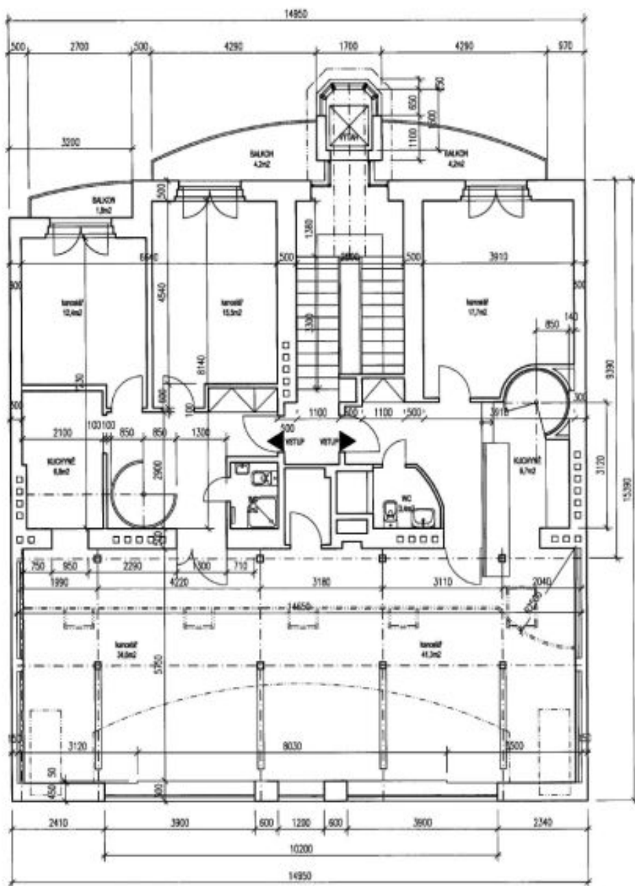
Půdorys 5.NP
