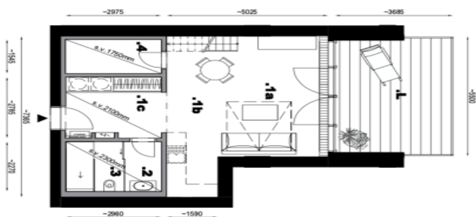
Úroveň Podlaží
