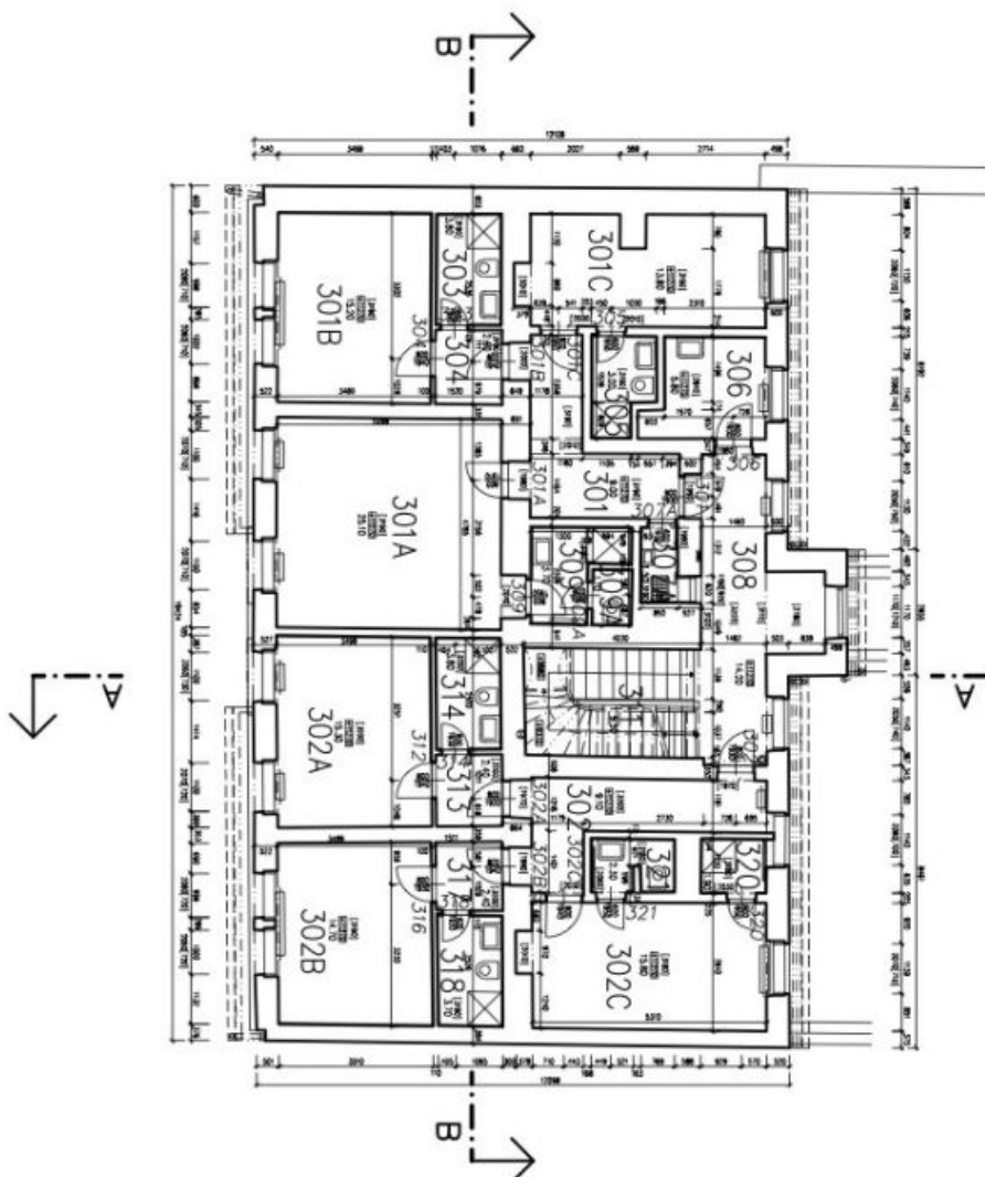
OBJEKT PENSION Hlinky 28a – půdorys III.patra 1:100
