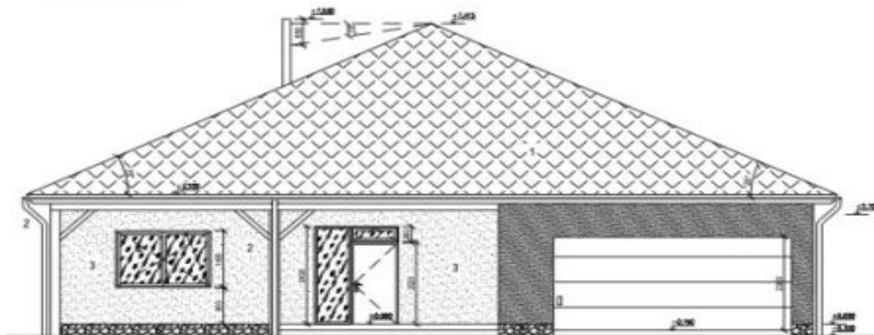
JIŽNÍ POHLED
