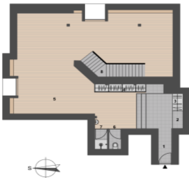
spodní podlaží / lower floor 110 m 2
