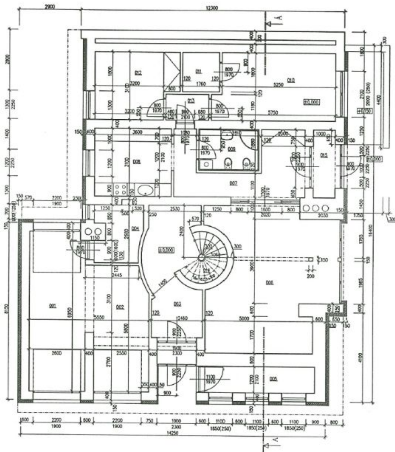
PŮDORYS I.PP
