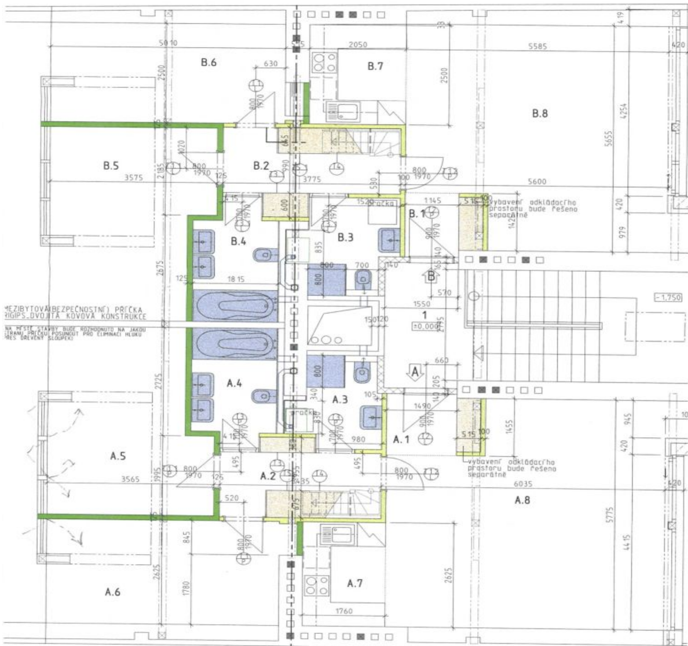
RYŠ PODKROVÍ, 1/50
