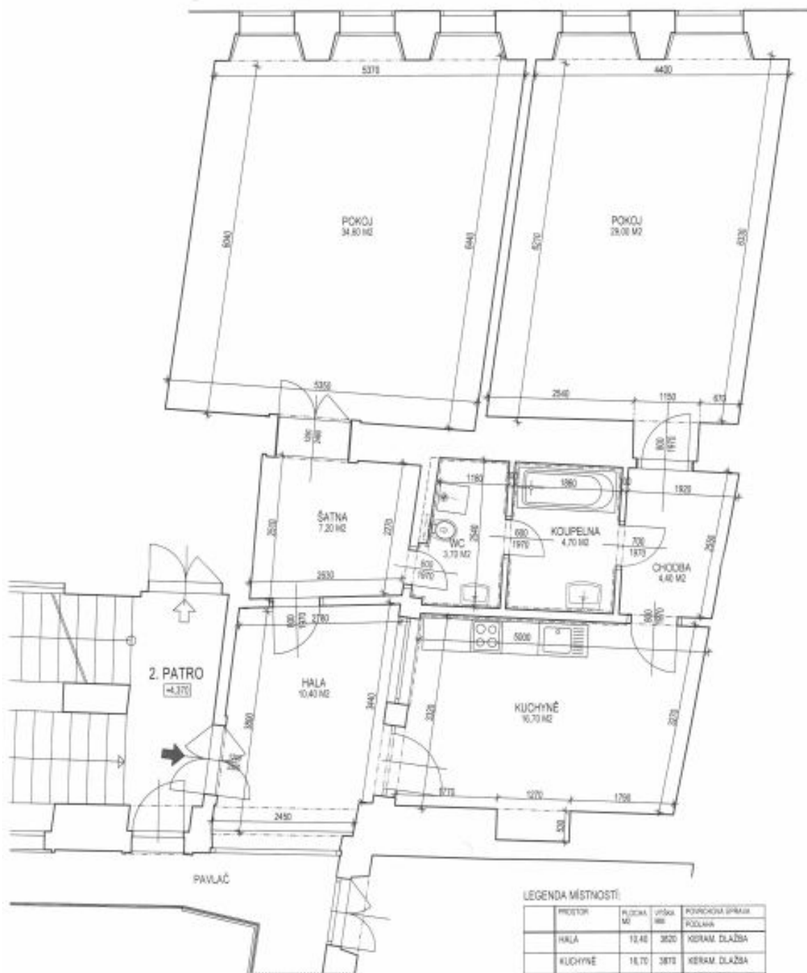
PŮDORYS BYTU - 2. PATRO ULIČNÍ TRAKT M 1:50
