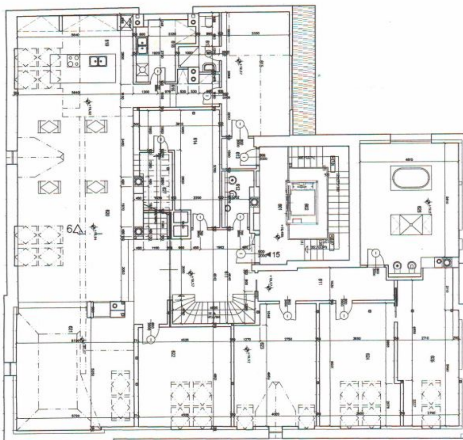
PUDORYS 6.N.P. 1:100
