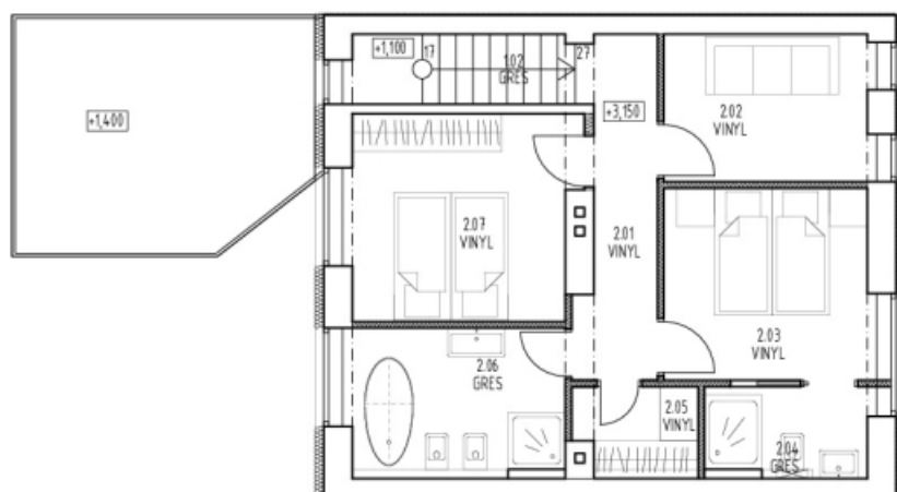
PÔDORYS 2.NP
