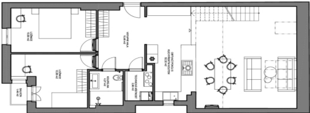
PŮDORYS 6.NP
