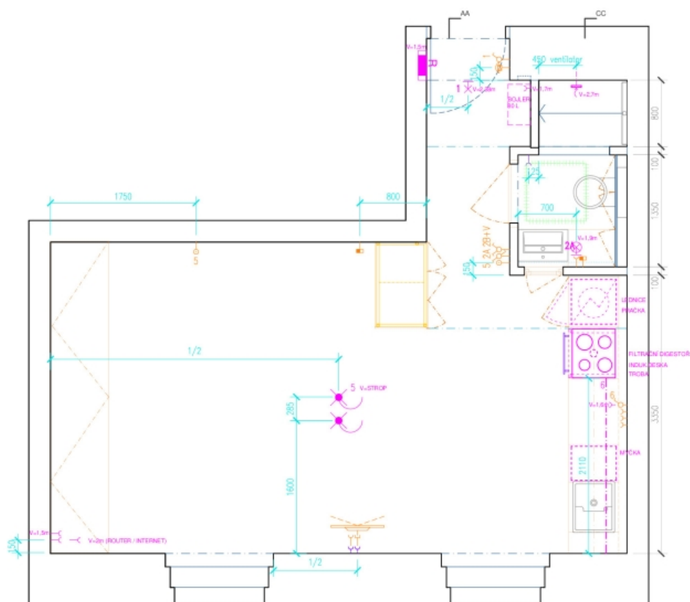
PŪDORYS BYTU
