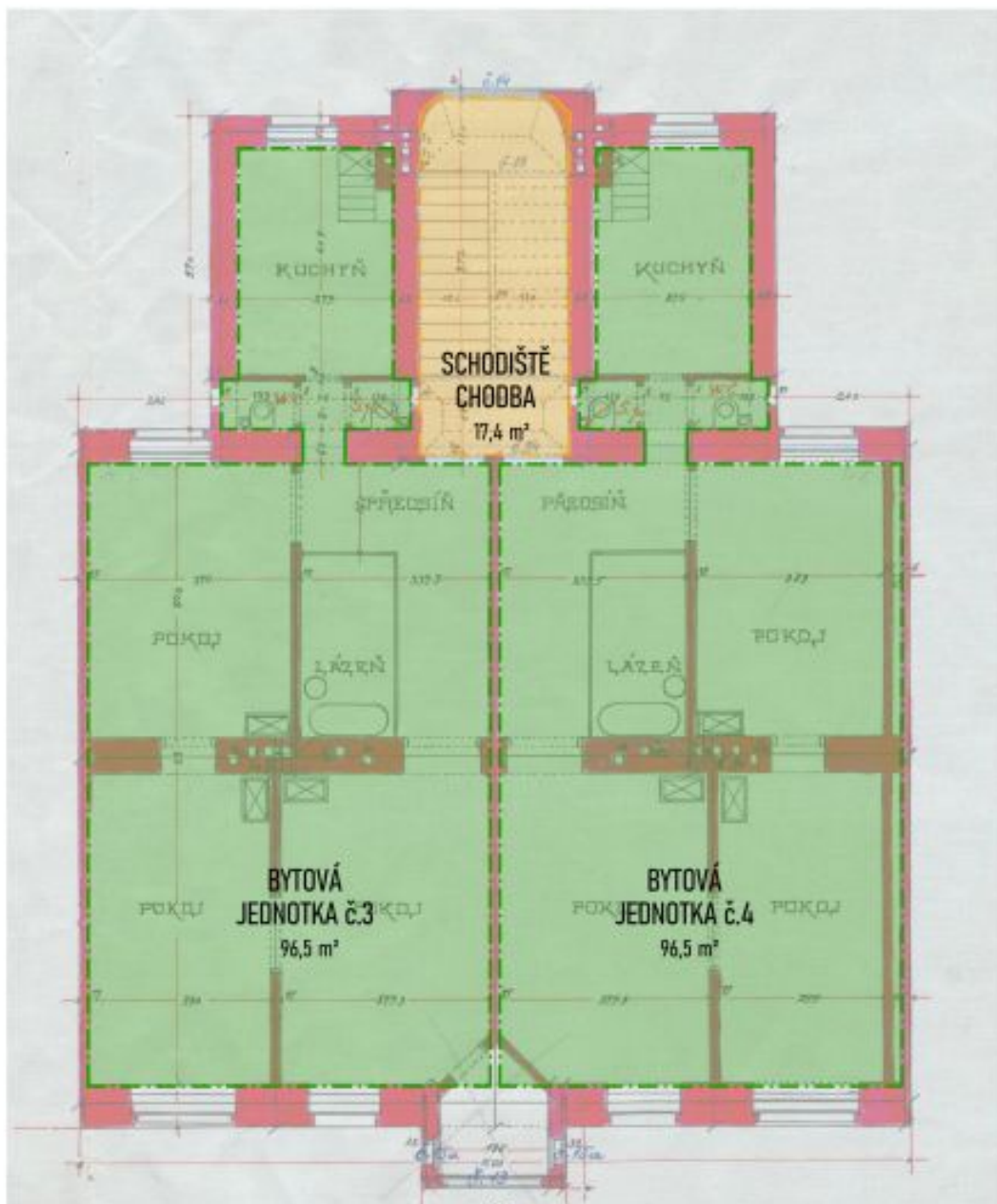
PŮDORYS 3.NP
