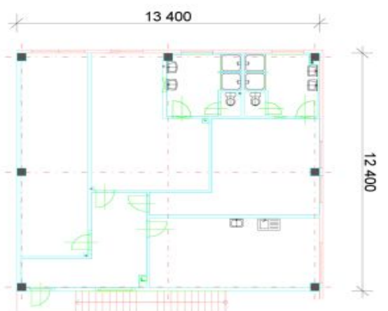
PŮDORYS 2.NP
