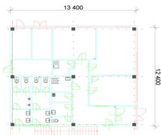
PŮDORYS 1.NP
