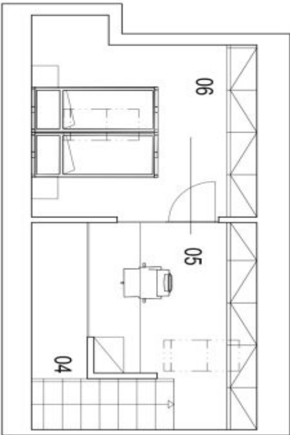
PŮDORYS 7.NP
