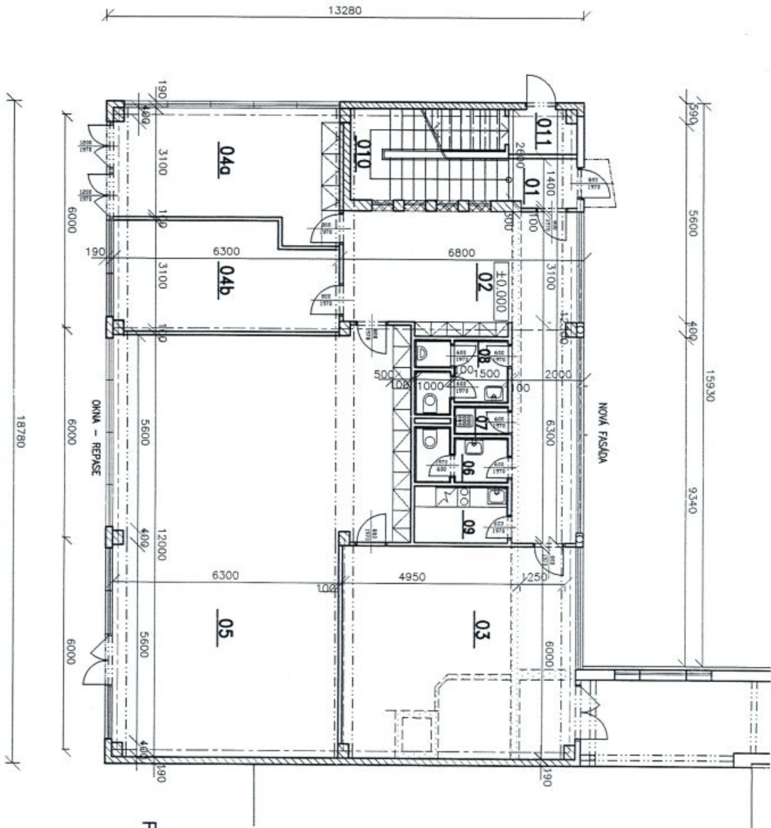
PŮDORYS 1.NP
