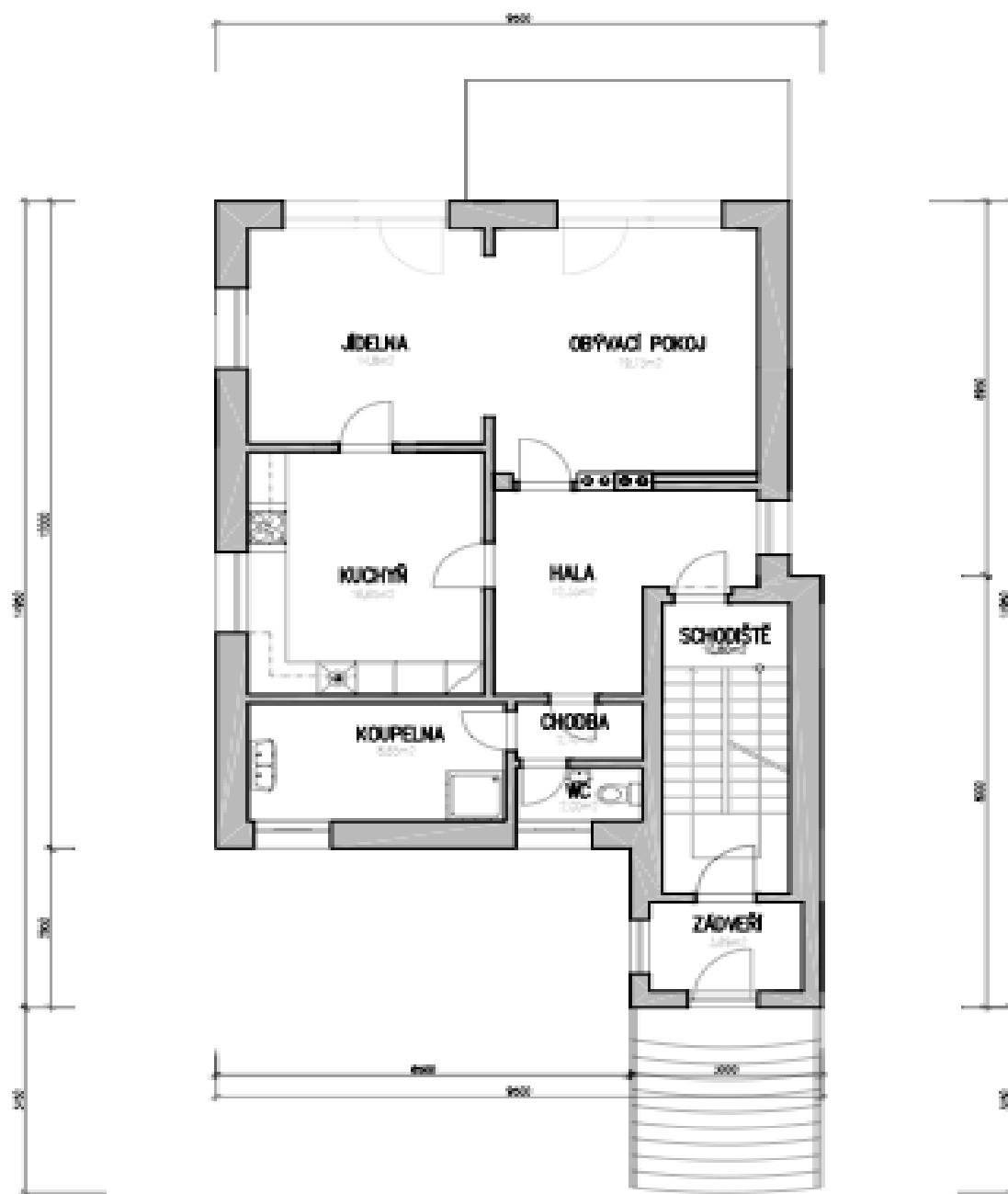
PŮDORYS 1.NP MĚŘ. 1:100
