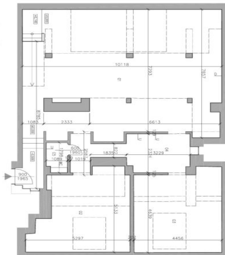
VSTUPNÍ PODLAŽÍ
