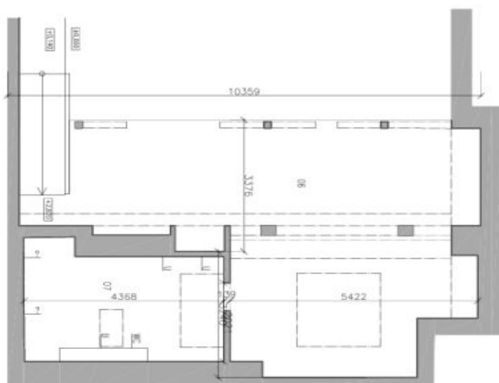
HORNÍ PODLAŽÍ
