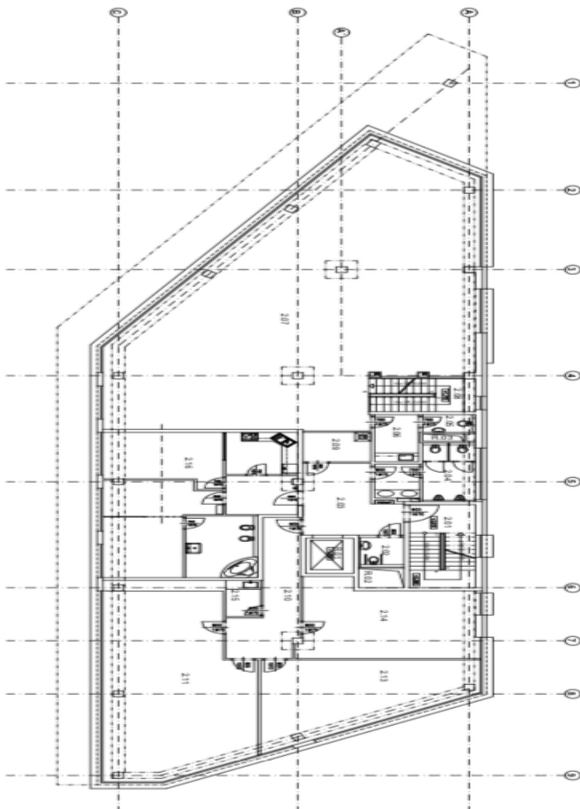
PŮDORYS 2.NP
