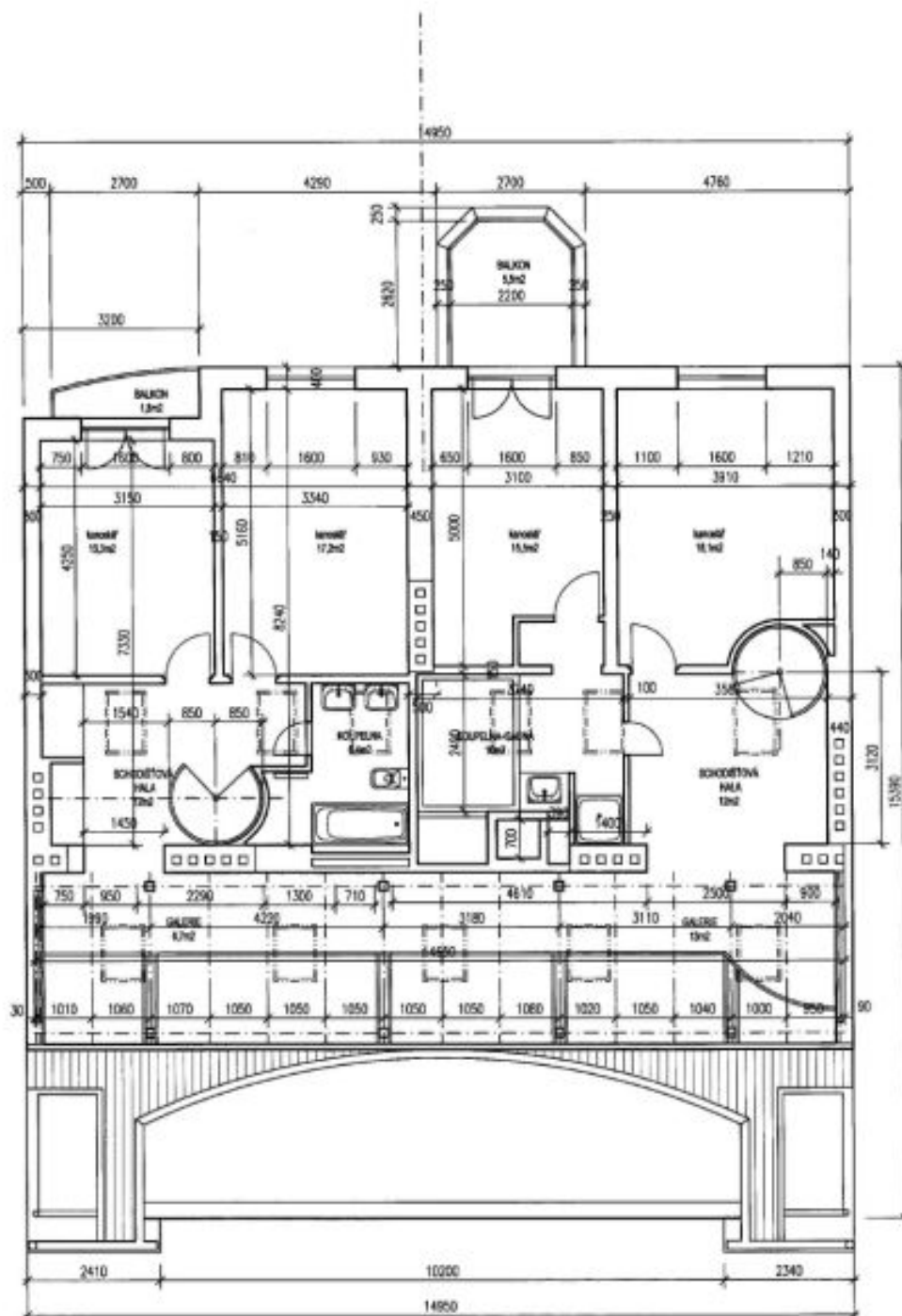
Půdorys 6.NP
