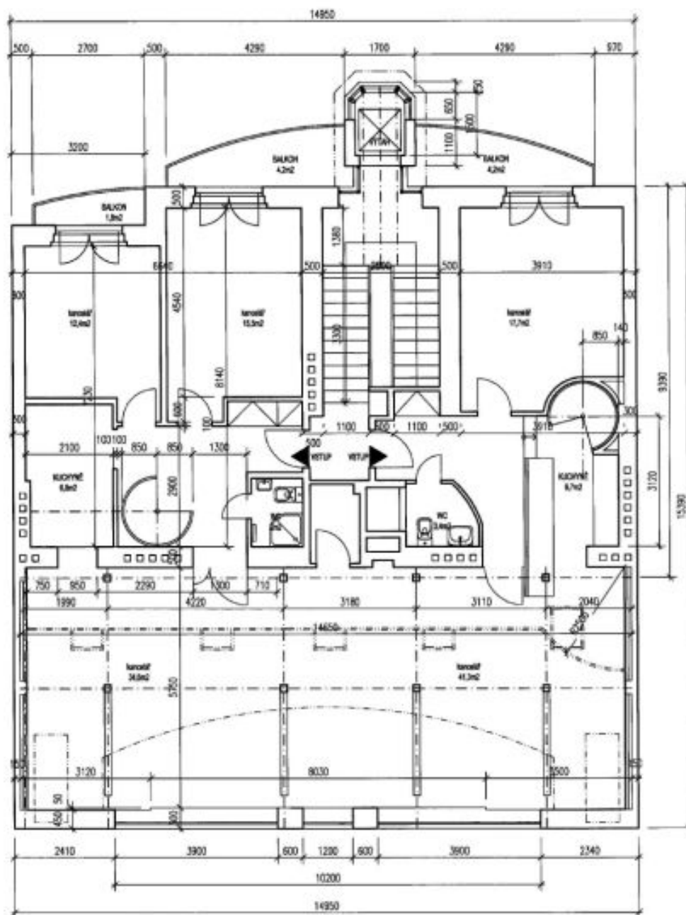
Půdorys 5.NP
