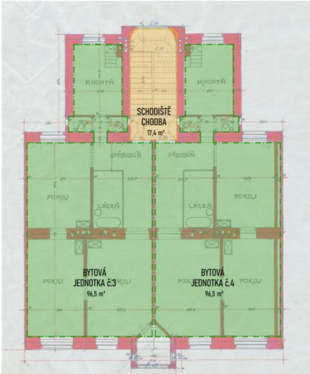
PŮDORYS 3.NP
